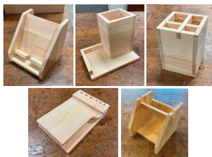
図4 市販の教材キットの製作例の試作 (上左から)①携帯端末ホルダ, ②小物立て[A], ③小物立て[B] (下左から)④メモホルダ, ⑤トイレーパーホルダ
